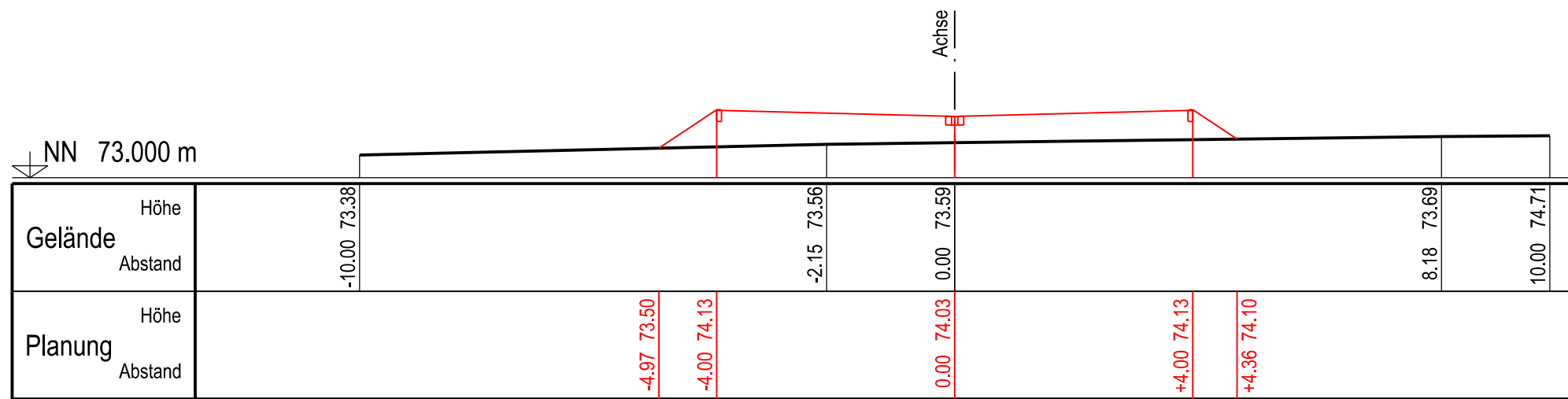
QP 6 - Planstraße B - 0+167,31
