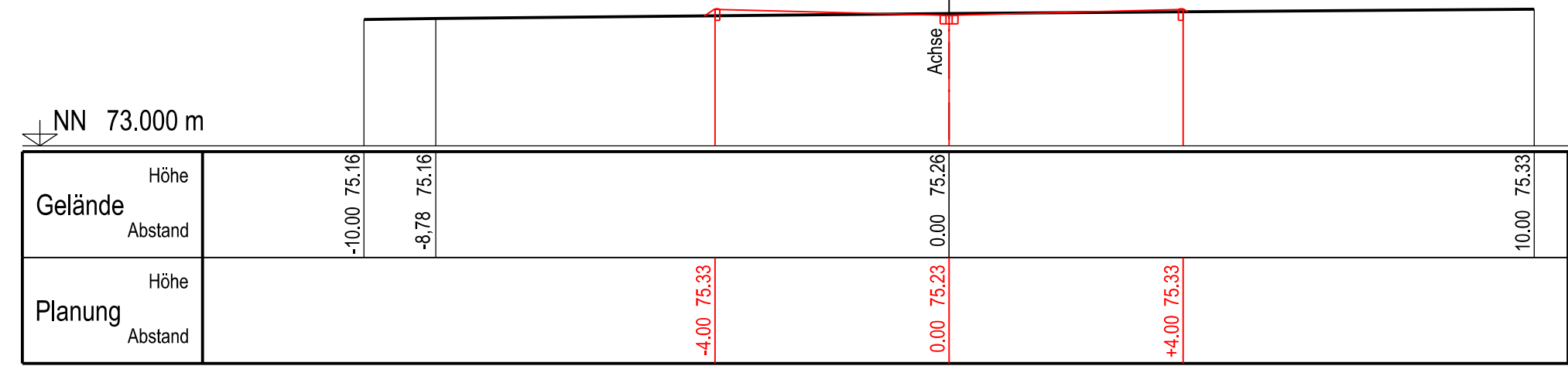
QP 2 - Planstraße B - 0+008.00
