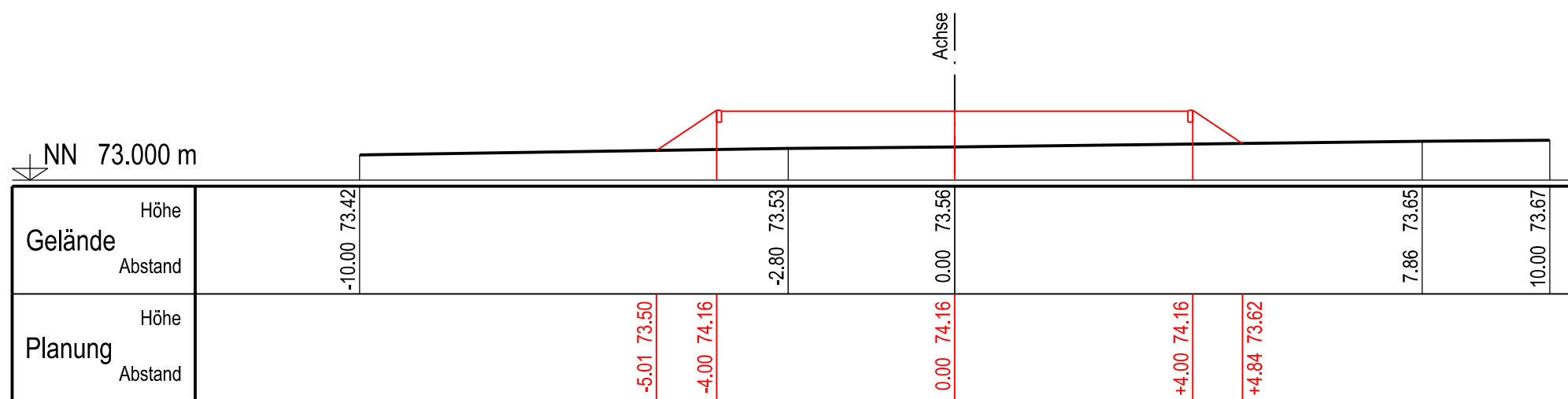
QP 7 - Planstraße B - 0+172,13
