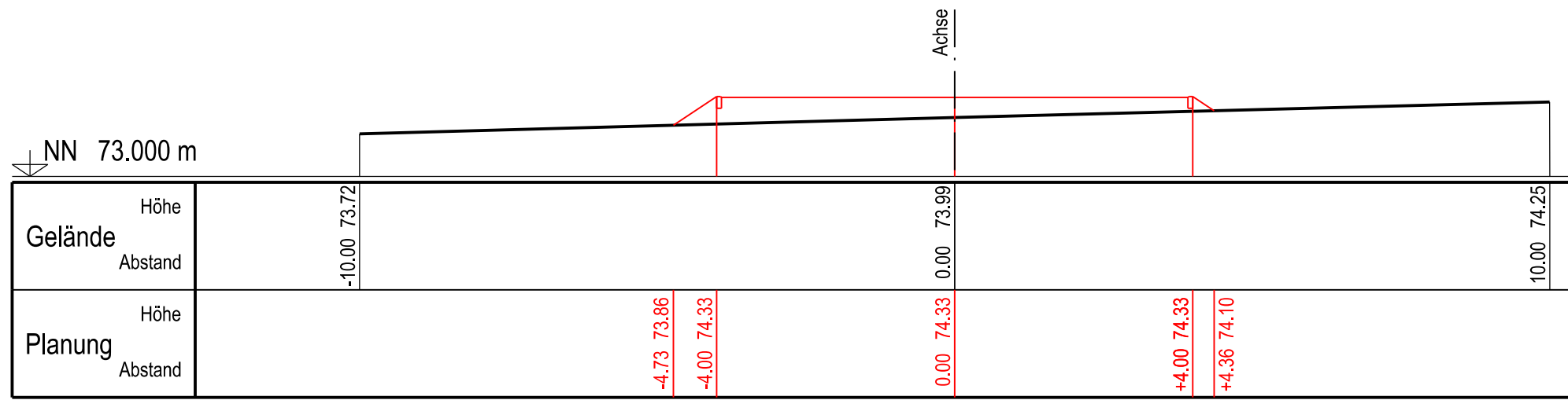
QP 5 - Planstraße B - 0+092,13
