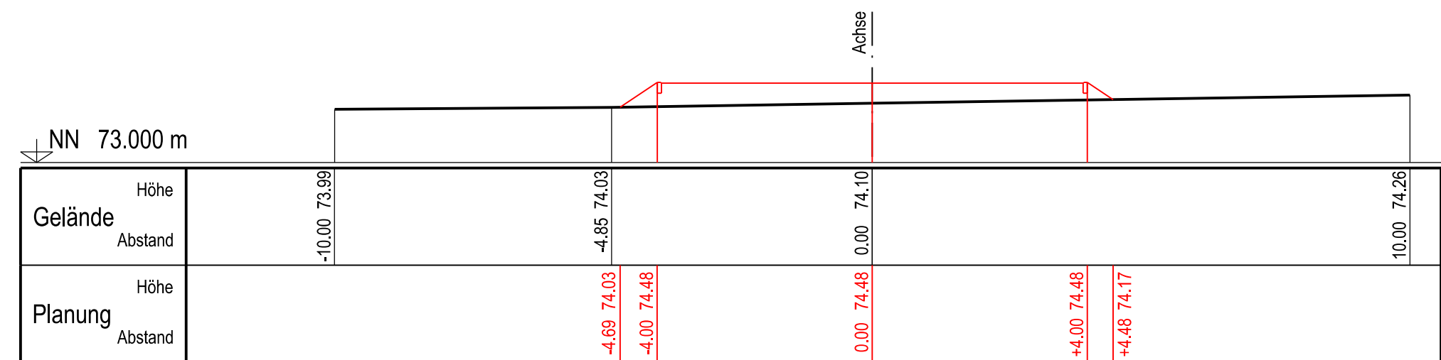
QP 4 - Planstraße B - 0+078.28
