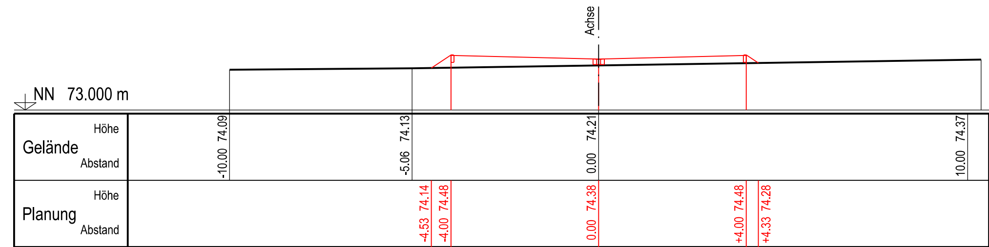
QP 3 - Planstraße B - 0+073.52
