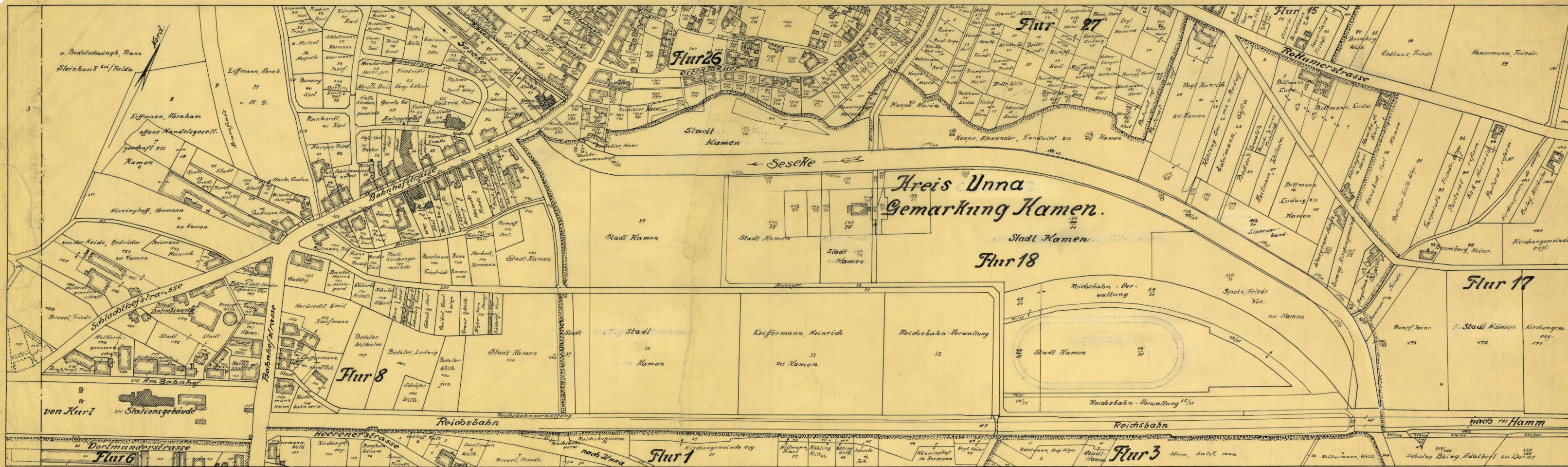
Fluchtlinienplan der Grünfläche K 2. Maßstab 1:2000.
